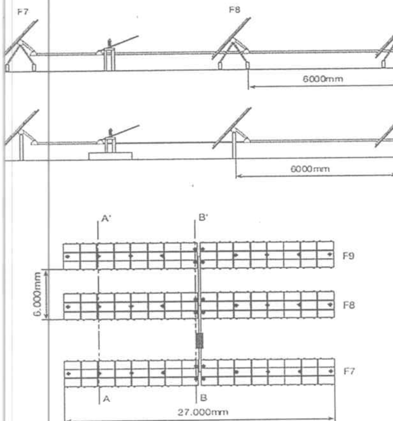
Figura N° 1. Dimensiones básicas de la estructura
